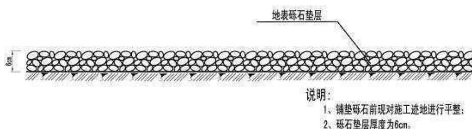
图 5.1-1 井场砾石压盖措施典型设计图
