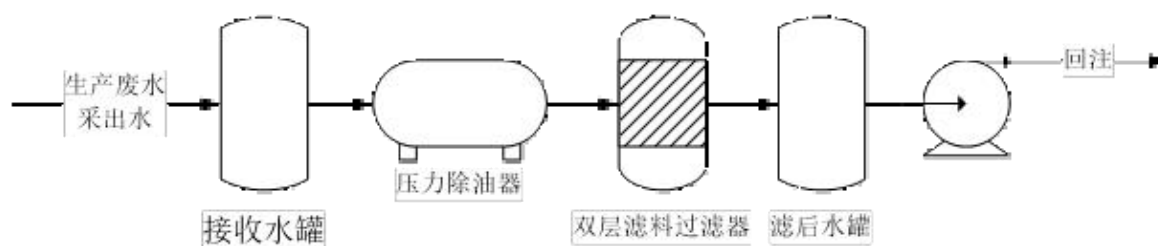
图 3.4-1 含油污水处理流程图
