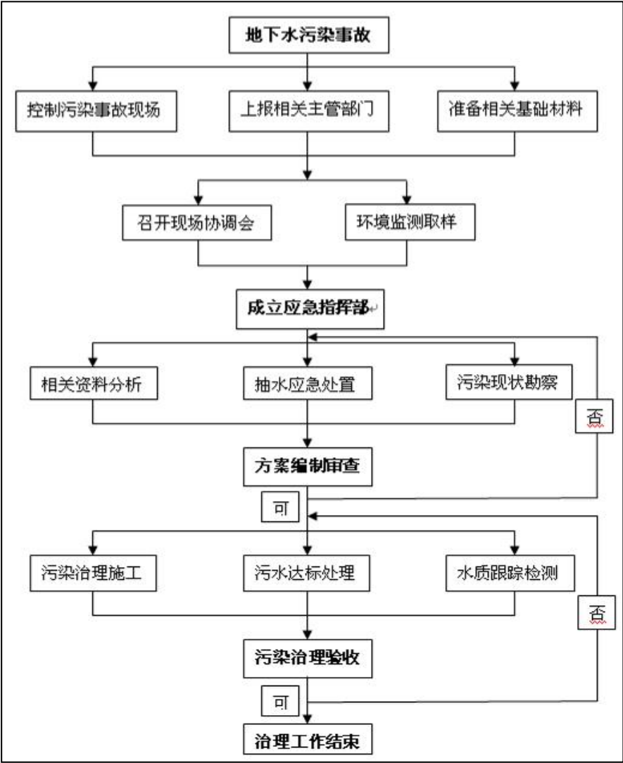
图 5.2-4 污染应急治理程序框图
